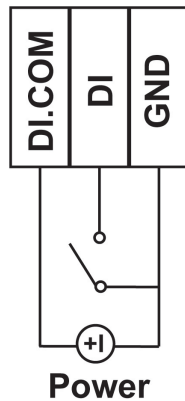
DI Dry Contact
